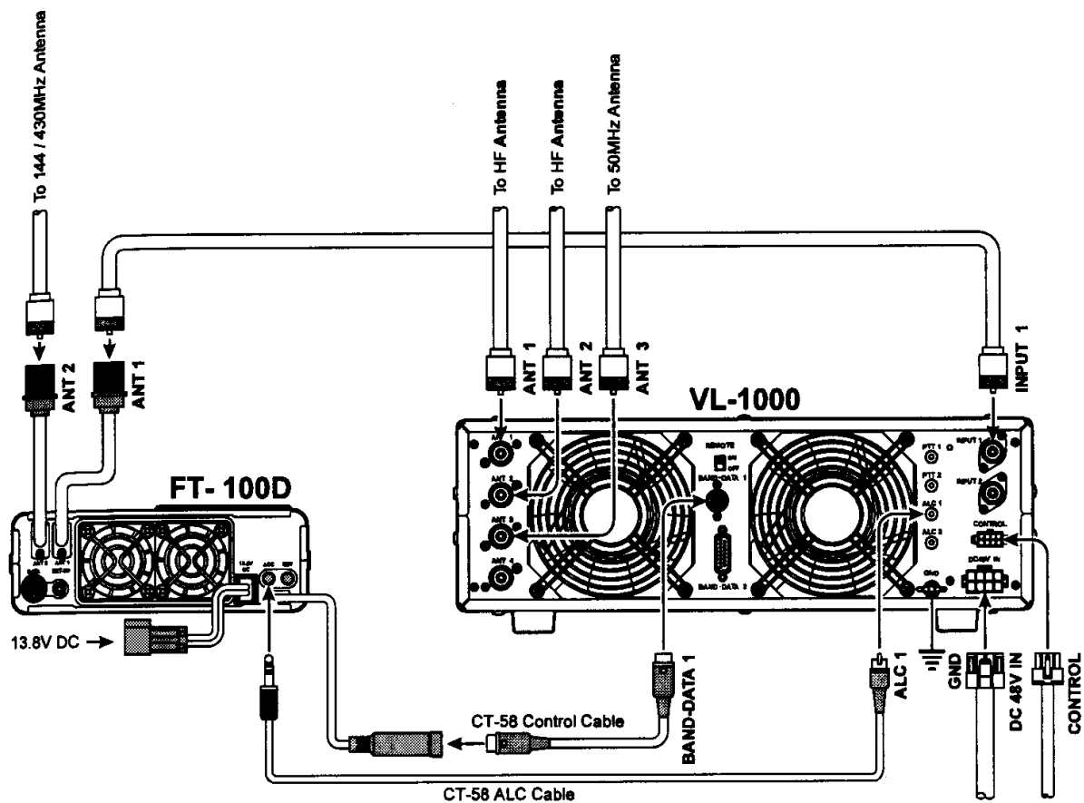
Schemat prawidłowego połączenia z wzmacniaczem.
